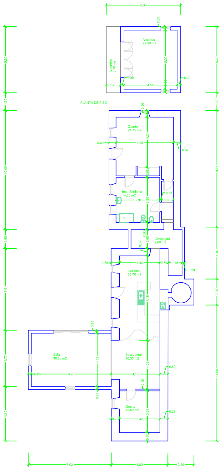
PLANTA DE PISO
