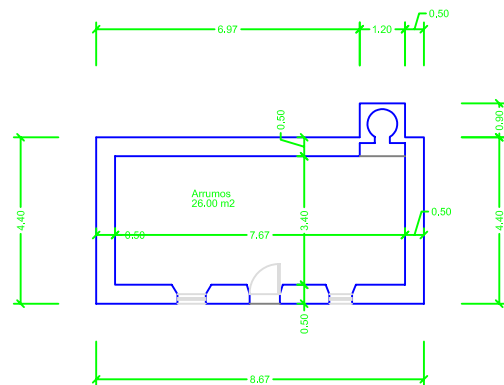
PLANTA DE PISO
